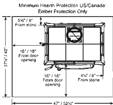
Right side load - 8023R
